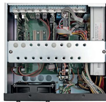
GO-083-10 Vista dall'alto senza copertura superiore
